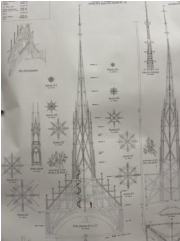
Caption: Plan de la flèche de Notre-Dame de Paris
